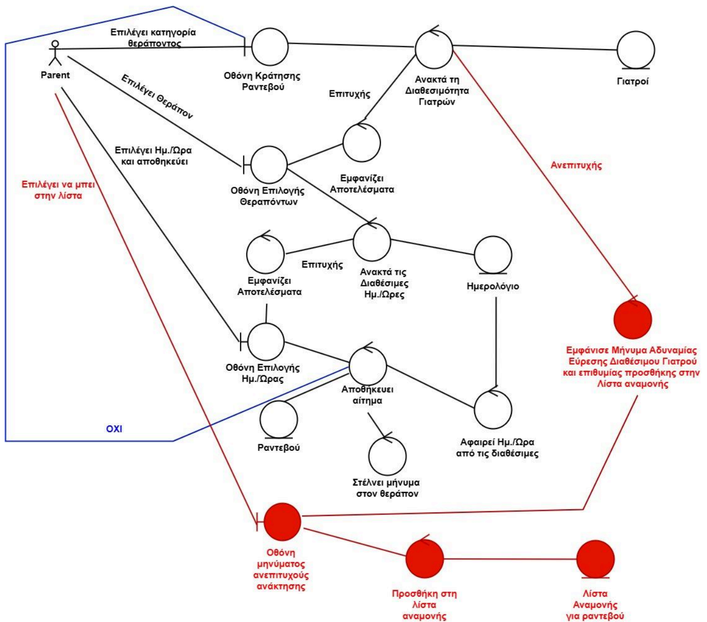
Robustness Diagram 1: Προγραμματισμός ραντεβού
