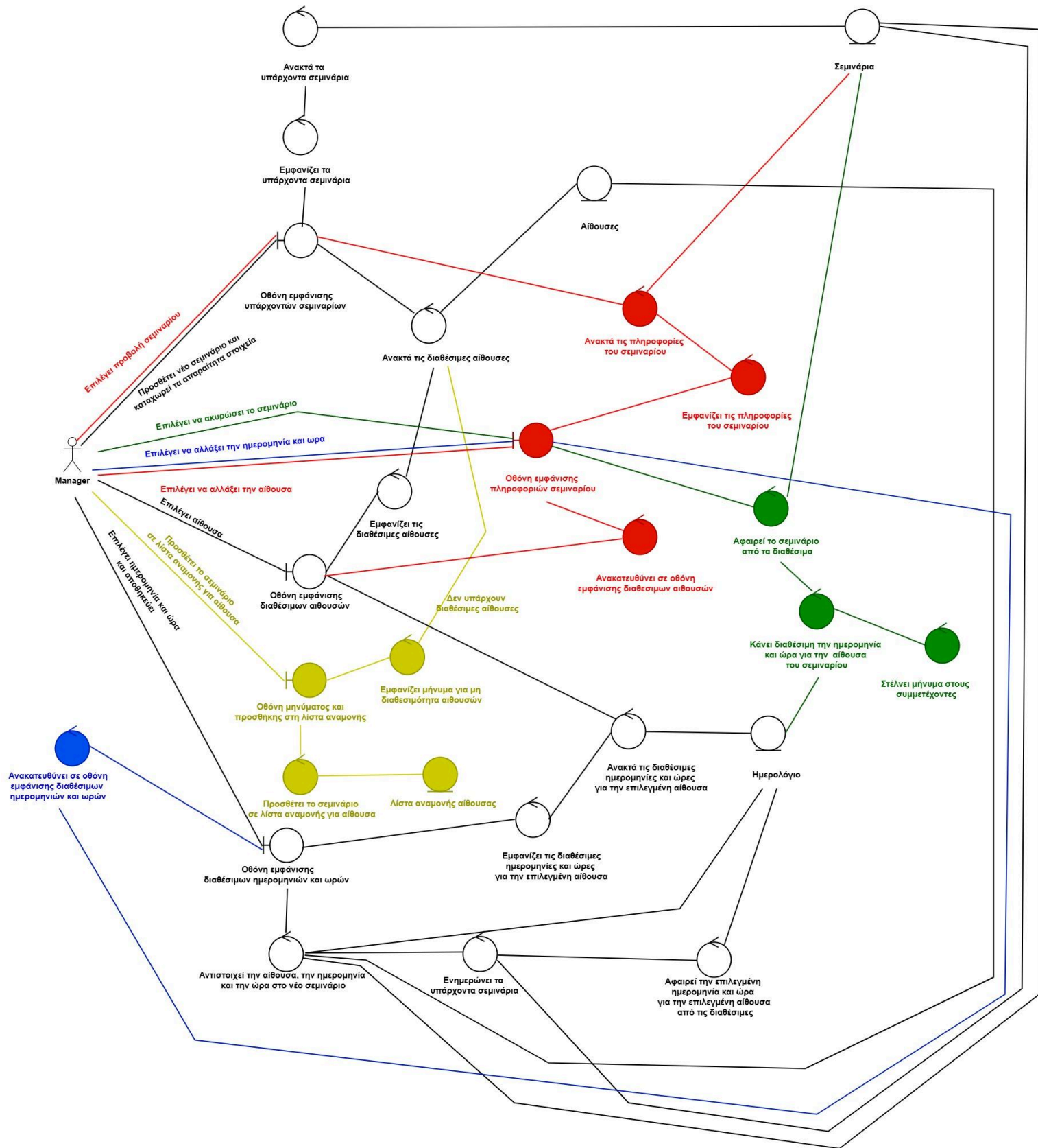
Robustness Diagram 5: Διαχείριση σεμιναρίων
