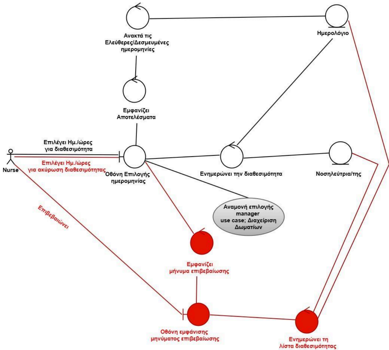
Robustness Diagram A: Δήλωση διαθεσιμότητας
