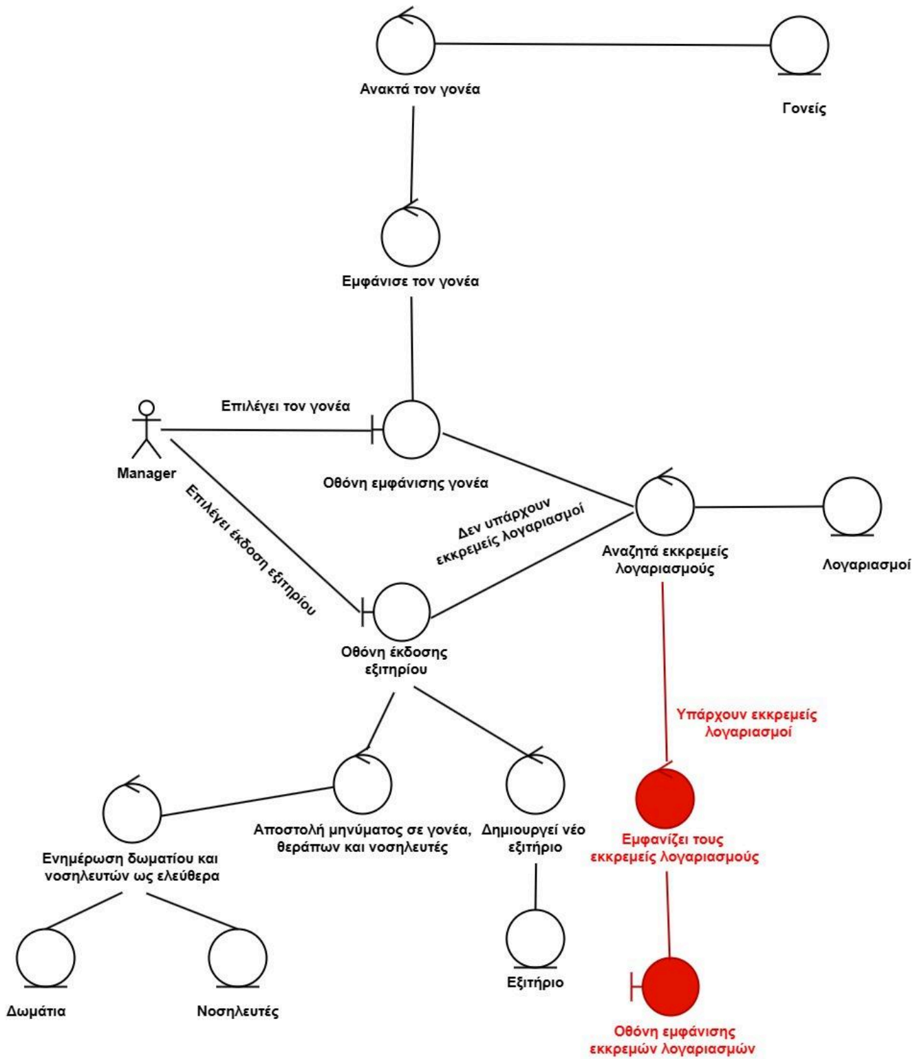
Robustness Diagram 6: Εκδοση εξιτηρίου
