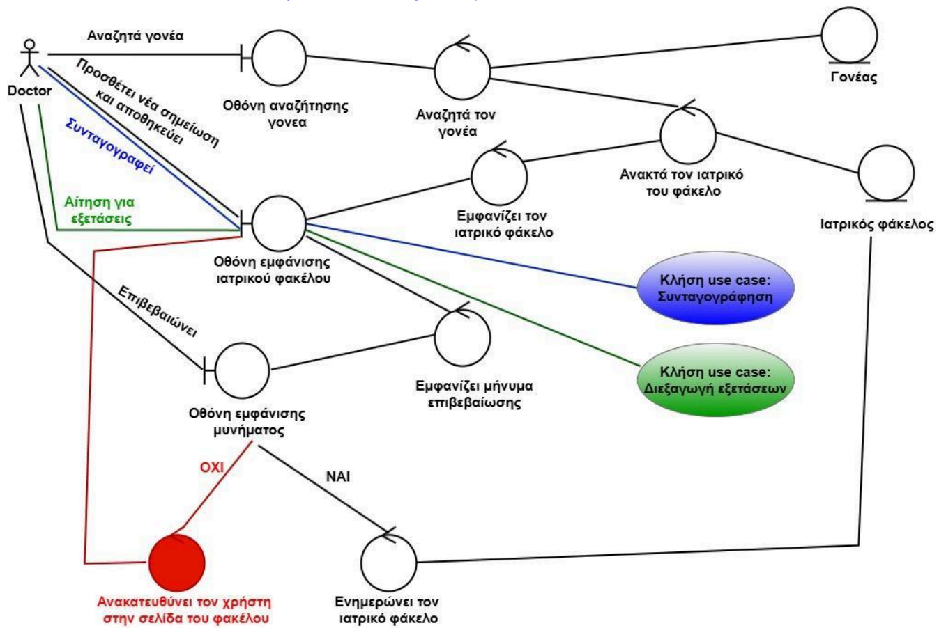
Robustness Diagram 8: Ενημέρωση ιατρικού φακέλου
