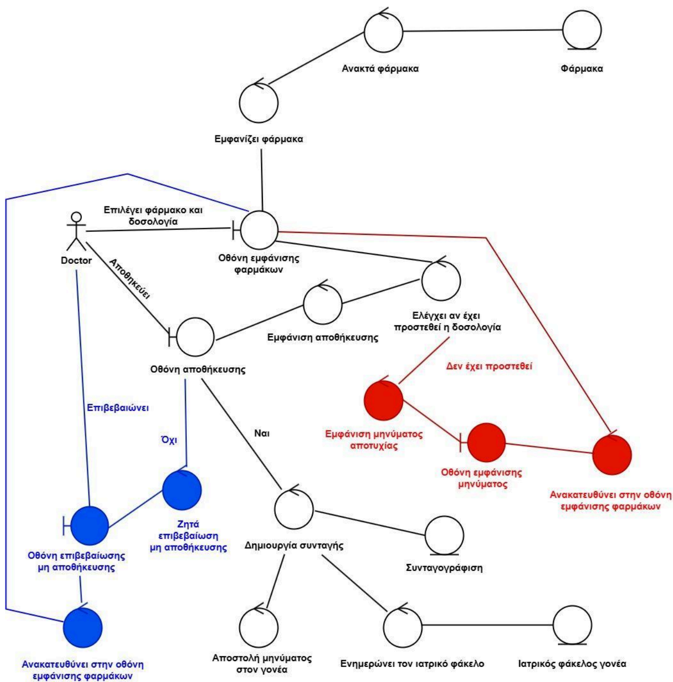
Robustness Diagram 9: Συνταγογράφηση
